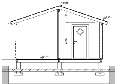
Leikkaus A-A 1:50
