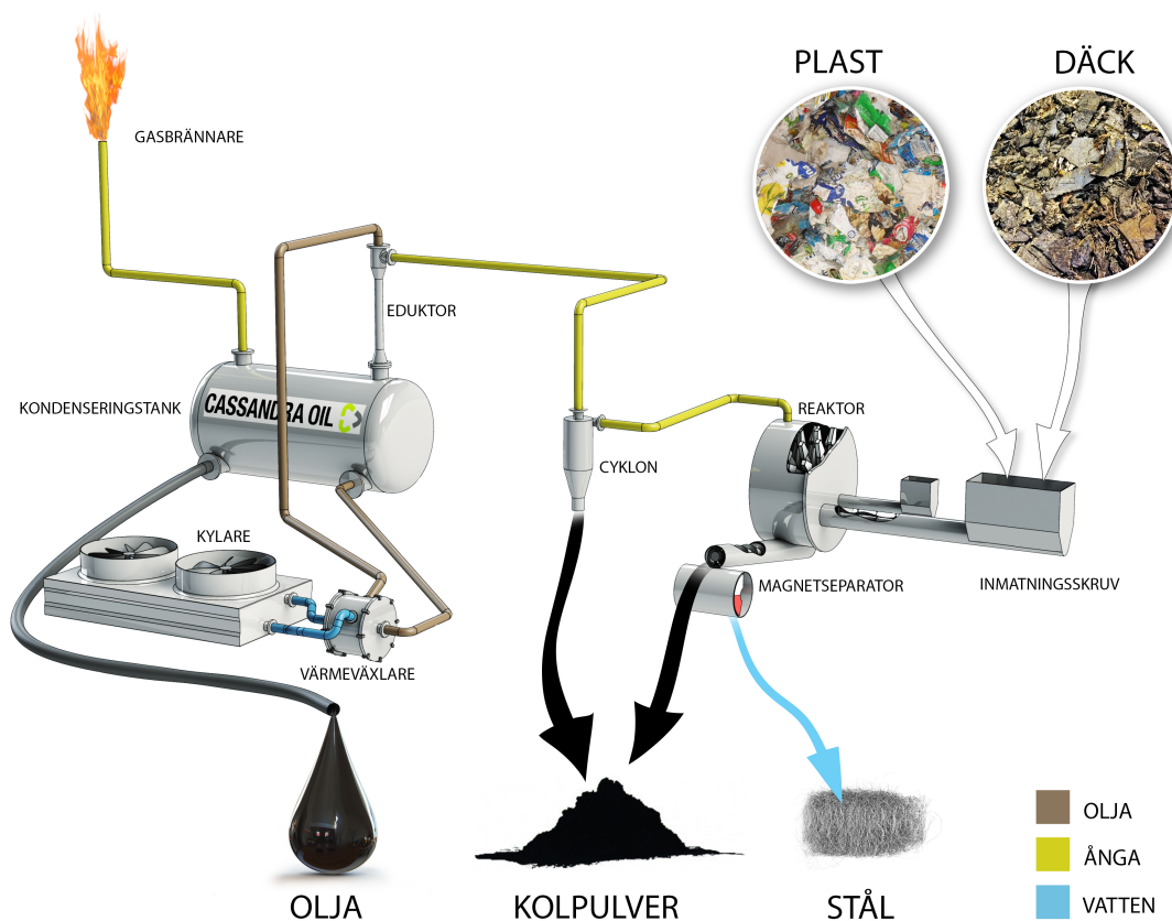
Bilden ovan visar materialflödet i en processanläggning
