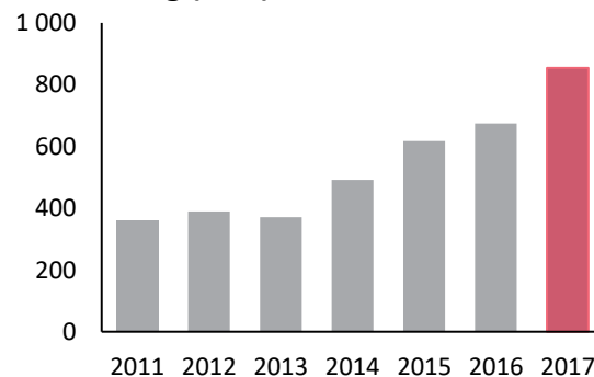
Omsättning (Mkr)
