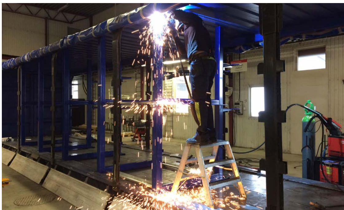
Svetsning av motorställ i en container till PWR BLOK, Mars 2018
