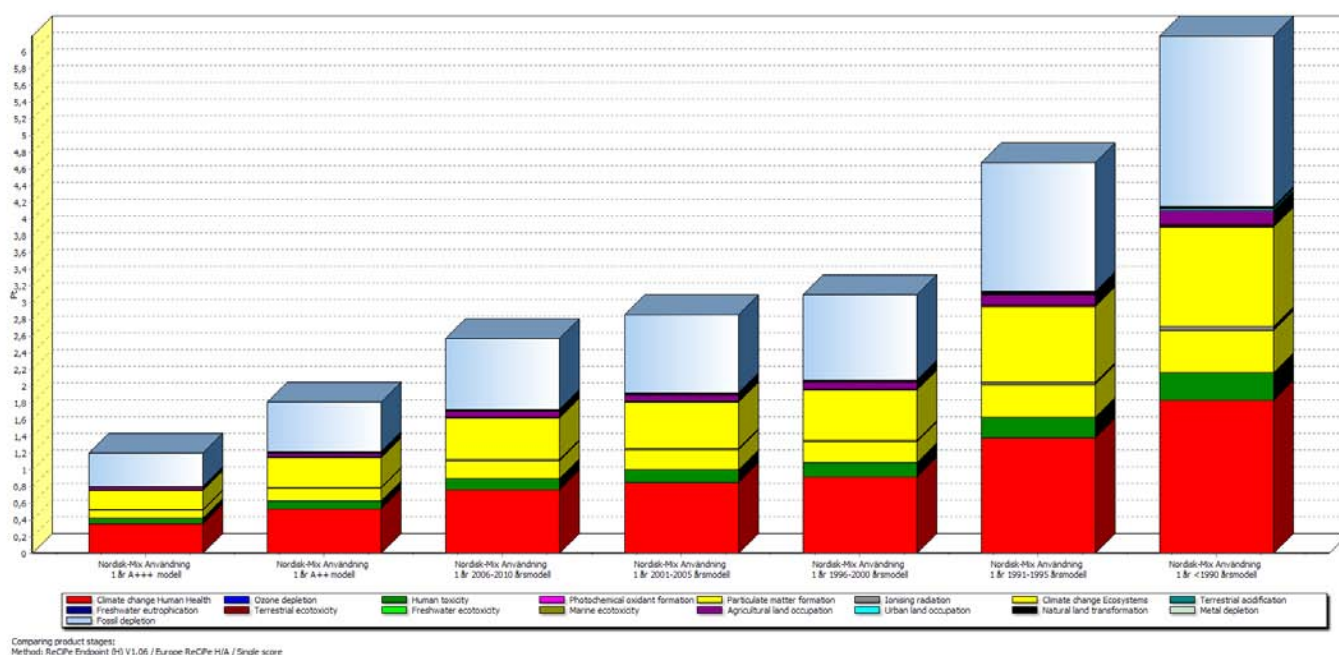
Figur 3. Resultat jämförelse miljöpåverkan för användning 1år av olika årsmodeller av kylskåp med nordisk elmix utvärderat med ReCiPe Endpoint (Pt).
