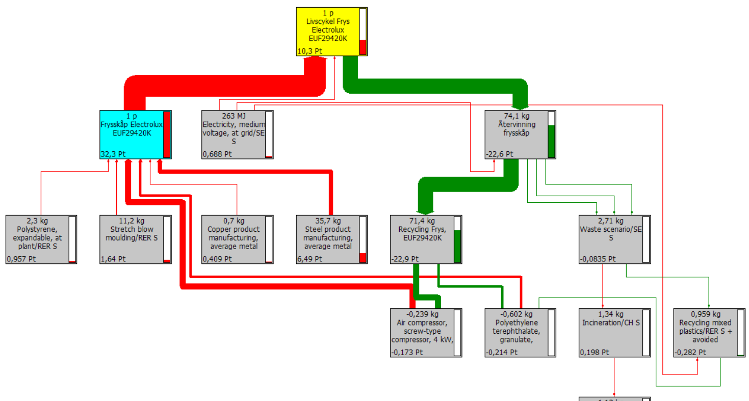
Figur 5. Nätverket visar vilka material och komponenter i livscykeln som har störst miljöpåverkan. Desto tjockare linje desto större påverkan. Bara de miljöaspekter som bidrar till den totala miljöeffekten med mer än 0,51 % visas i nätverket.
