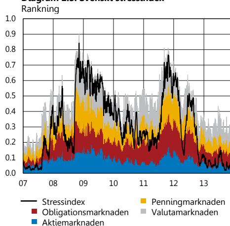
Diagram 2:3. Svenskt stressindex
