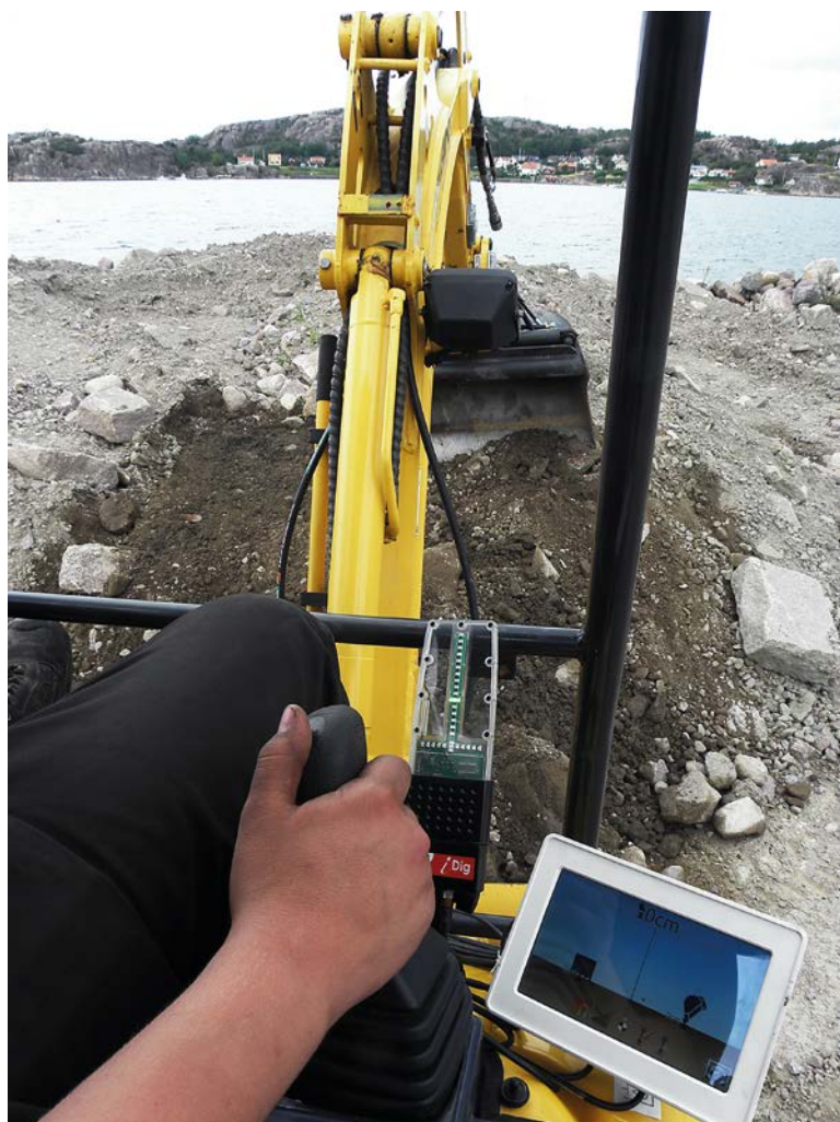
Grävsystemet iDig 2D Touch monterat på minigrävaren Abelco XC18srE.
